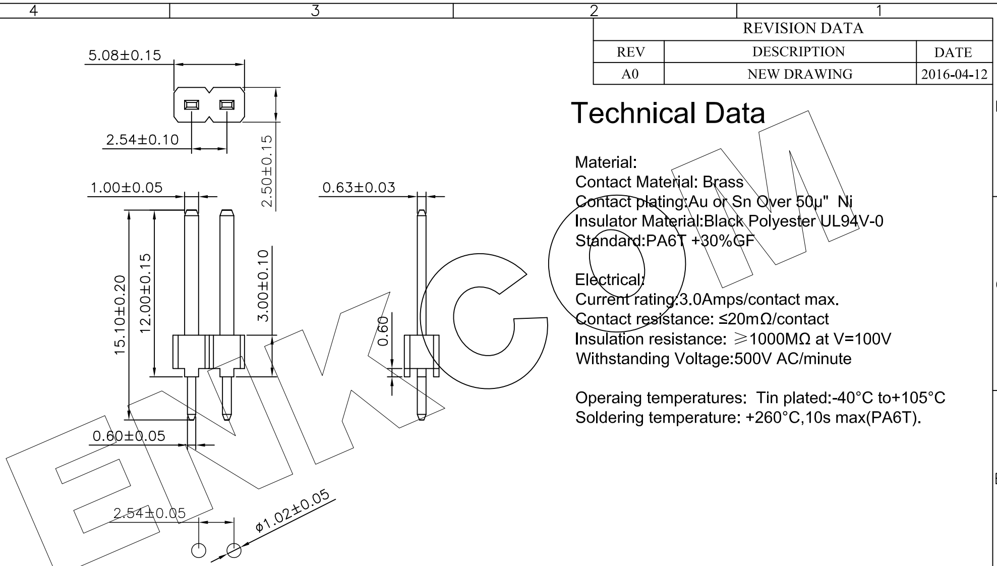
P.C.B LAYOUT
