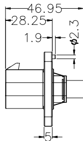
插座
