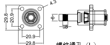
螺纹通孔 (L)
