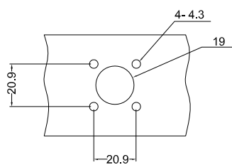
面板开孔尺寸
