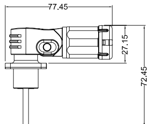
闭合状态
