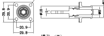
通孔 (T)
